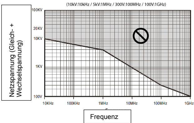
Figure 5: Derating / Herabgestufte Spannungskurve
