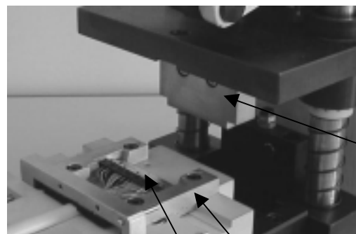
プラグサブアセンブリ Plug sub-assembly
